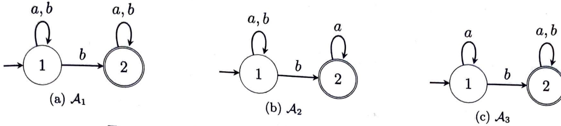
FIGURE 1 – Trois automates reconnaissant le même langage
